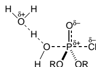
3 R = aryl
